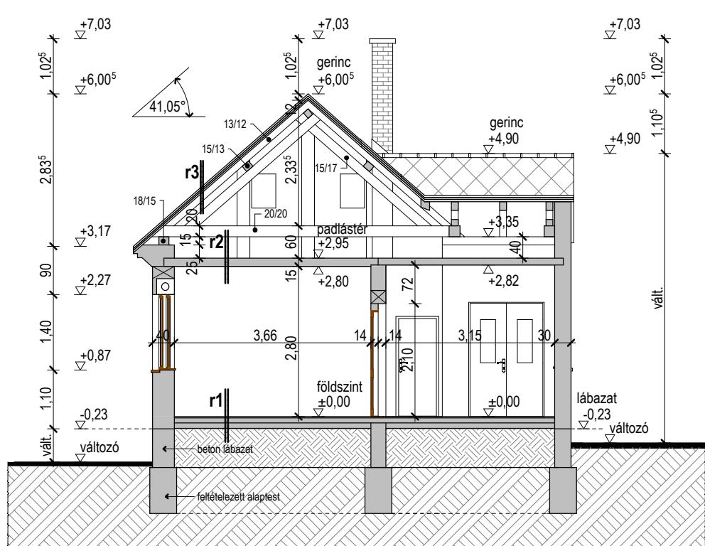
FELMÉRÉSI A-A METSZET M 1:100
