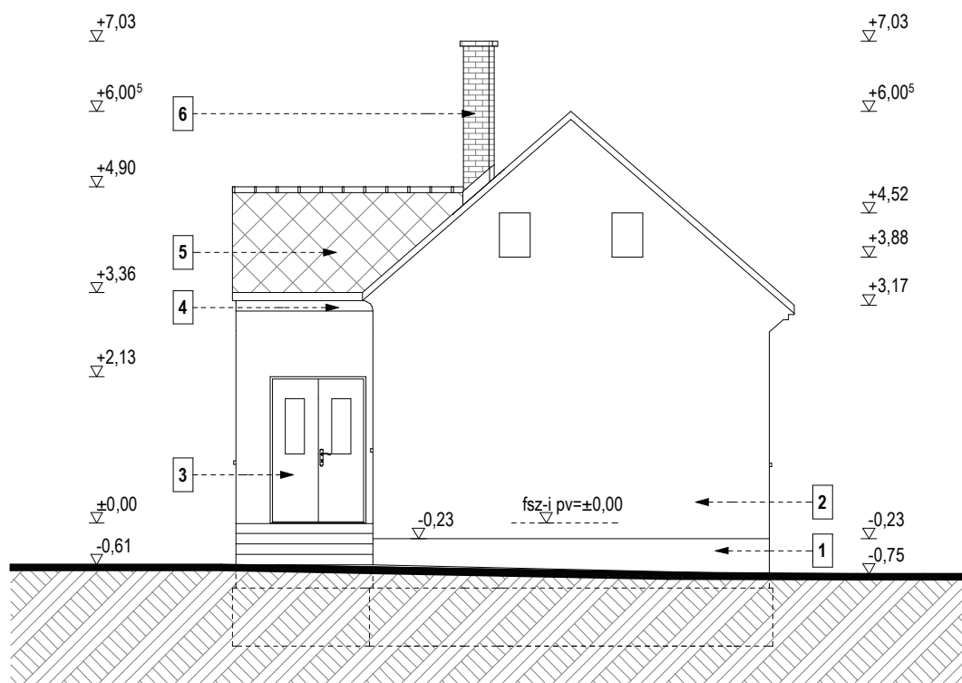
FELMÉRÉSI DÉLI HOMLOKZAT M 1:100
