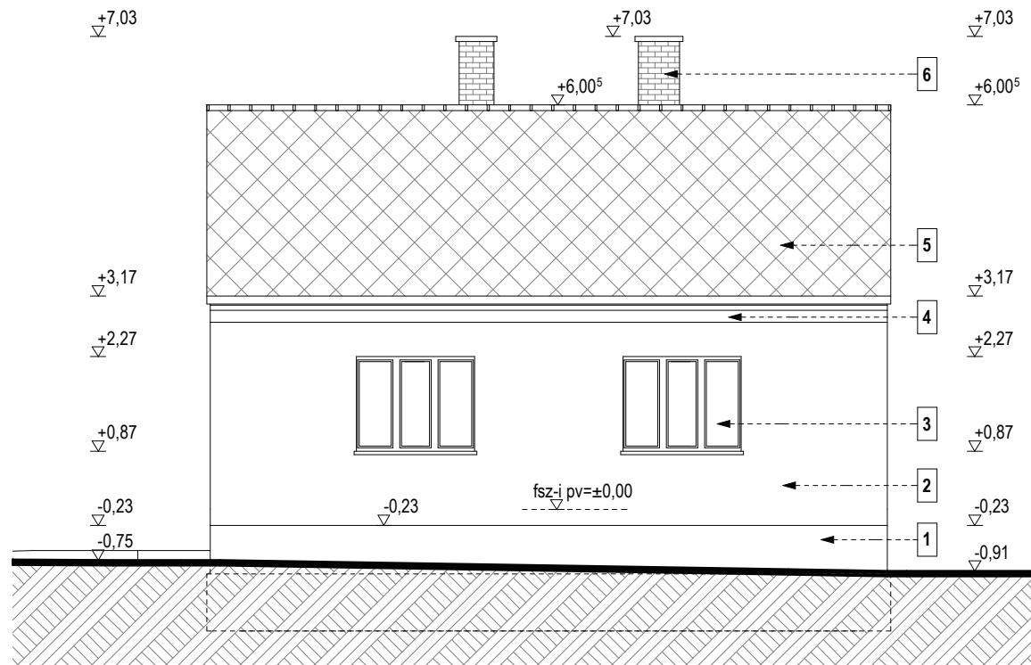
FELMÉRÉSI KELETI HOMLOKZAT M 1:100
