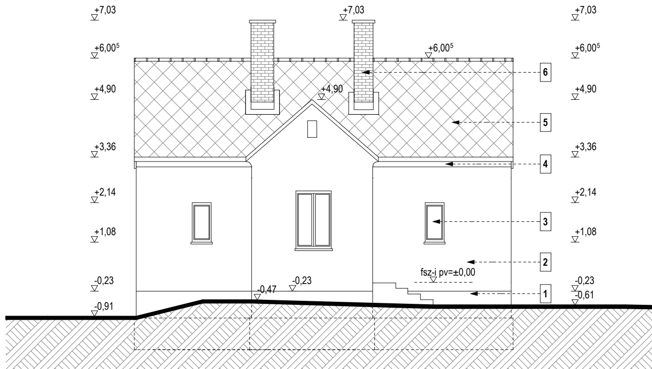
FELMÉRÉSI NYUGATI HOMLOKZAT M 1:100
