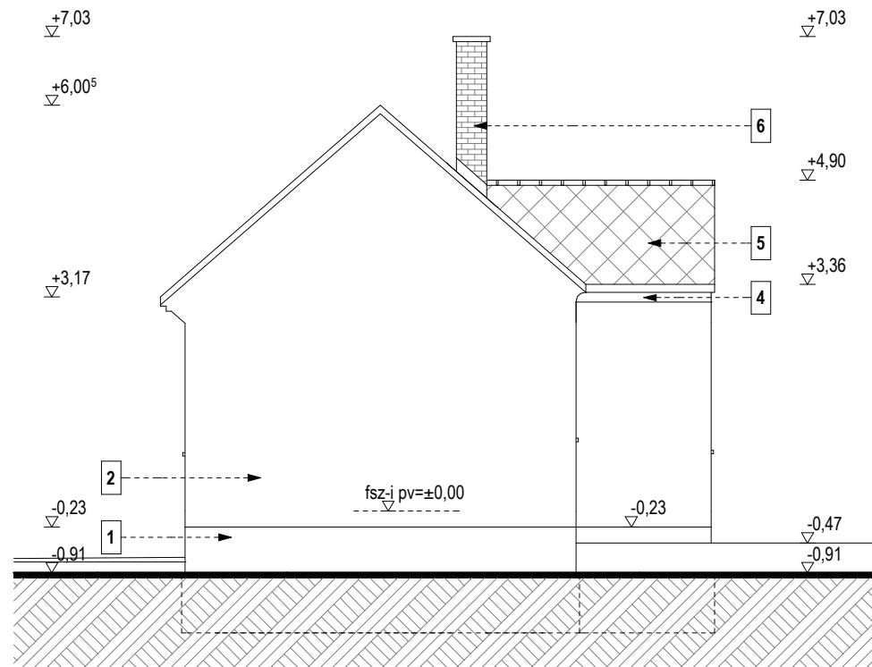
FELMÉRÉSI ÉSZAKI HOMLOKZAT M 1:100
