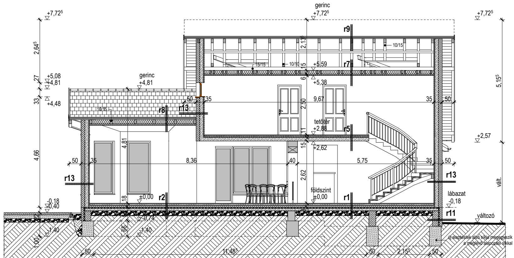
TERVEZETT B-B METSZET M 1:100
